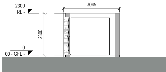
8 Section A-A 1:100
